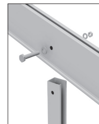
Detalle de la conexión - Balsas
