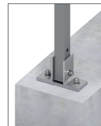
Placas de pie con anclajes fijos
