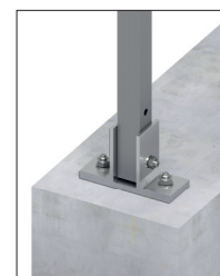
Fußplatten mit Befestigungsanker
