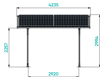
Vorderansicht
