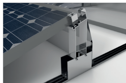
Vista detallada del soporte trasero
