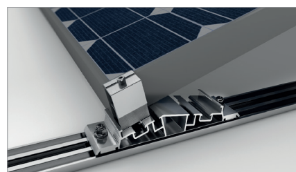
Vista detallada del pie delantero
