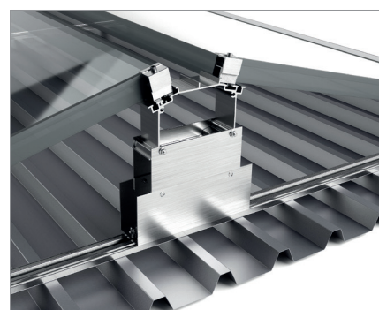
Wspornik środkowy
