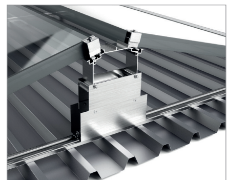
Soporte trasero
