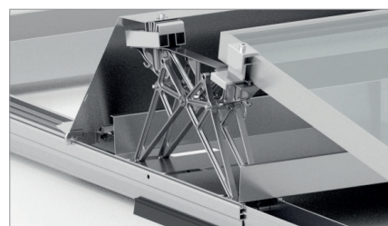
Tylna podpora 10°
