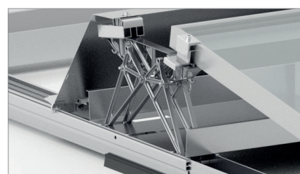
Achterste steun 10°
