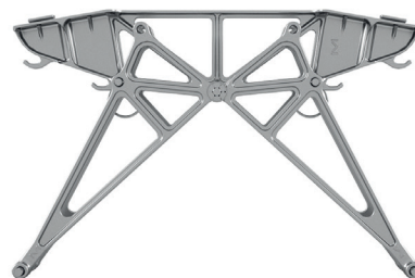
Suport central de 10° pentru orientare est/vest
