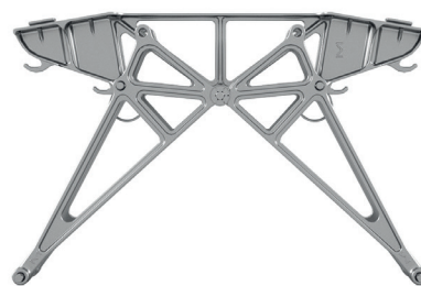
Środkowa podpora 10°
