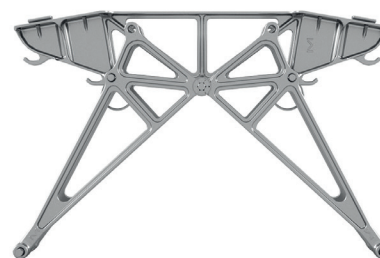
Middel steun 10° voor oost-west oriëntatie
