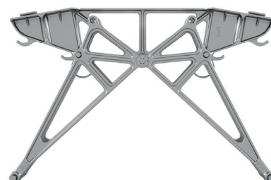
Középső támasz 10° kelet/nyugati tájoláshoz
