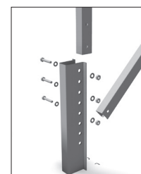
Dettaglio della connessione palo
