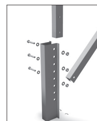
Détail de connexion poteau
