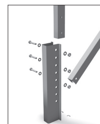
Detalle de la conexión - Postes
