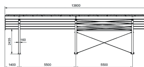
Vista frontale
