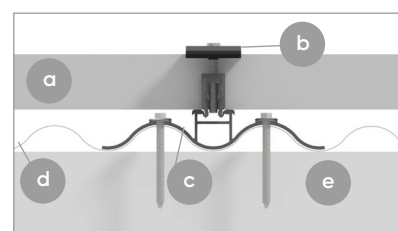
Horizontale snede, dwarsuitvoering
