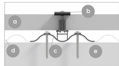
Horizontaler Schnitt, Quermontage
