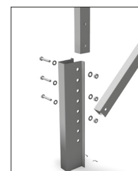
Detail spojů konzoly
