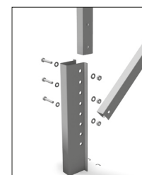
Details van verbinding: paal
