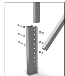
Détail de connexion poteau
