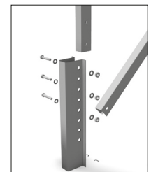
Detalle de la conexión - Postes
