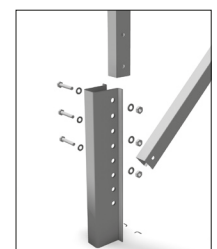
Anschlussdetail Pfosten
