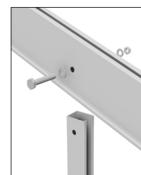
Anschlussdetail Stütze- Sparren
