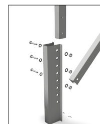
Detail spojení nohy a příčniku
