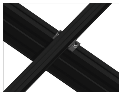
Mocowanie elementu skośnego do podpory
