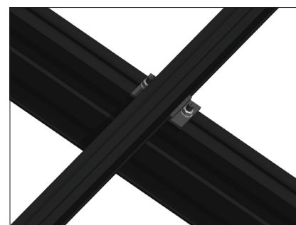
Dettaglio della connessione Supporto - rafter
