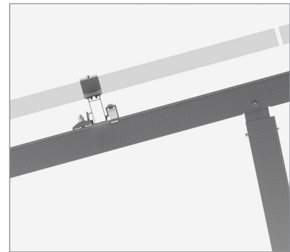
Zijaanzicht opbouw
