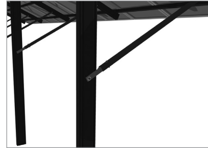
Anbindung der Diagonale an den C-Pfosten
